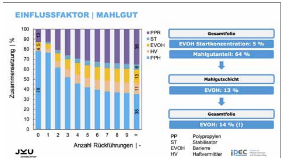
Einflussfaktoren auf die Zusammensetzung des im Kreislauf rückgeführten Mahlgutes.
